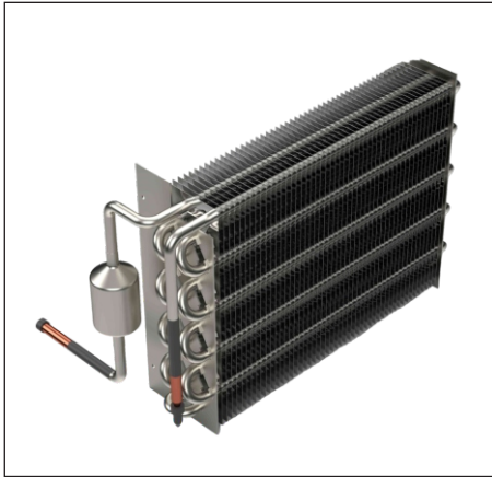
FROST FREE EVAPORATOR
